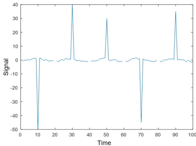
Chýbajúce a odľahlé dáta
