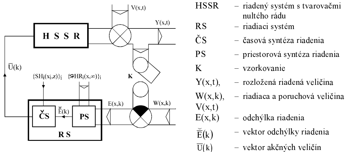
Obr. 3 Riadiaci obvod s rozloženými parametrami
