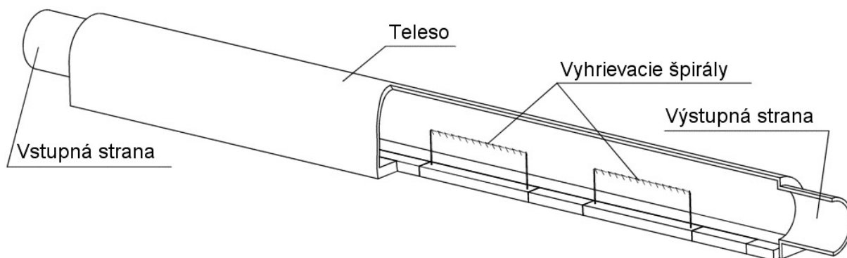
Obr 3. Trojrozmerný model vyšetřovanej teplovzdušnej sústavy s rozloženými parametrami
