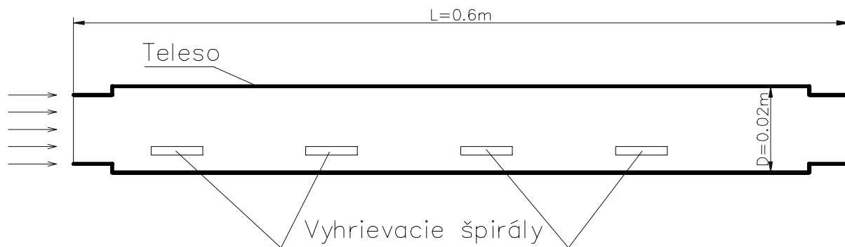
Obr 4. Zjednodušený dvojrozmerný model teplovzdušnej sústavy s rozloženými parametrami
