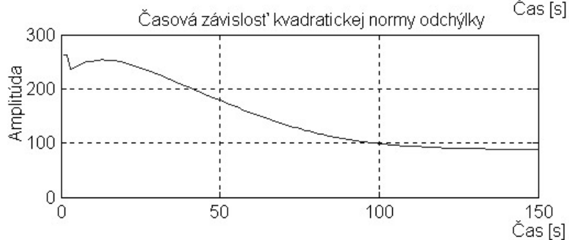
Obr 6. Proces riadenia teplovzdušného systému s rozloženými parametrami pre skokovú rozloženú žiadanú veličinu v prostredí MATLAB - FEMLAB
